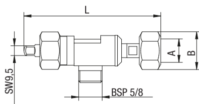
Hilfsventil mit Überwurfmutter
